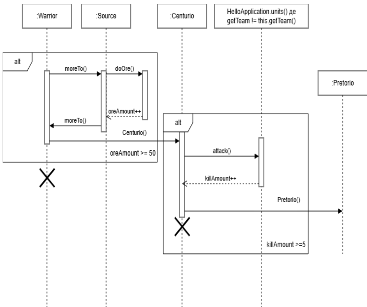
Рисунок 3.6 – Діаграма послідовності
