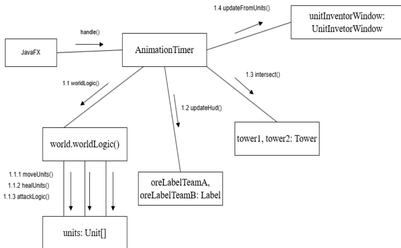
Рисунок 3.5 – Діаграма кооперації
