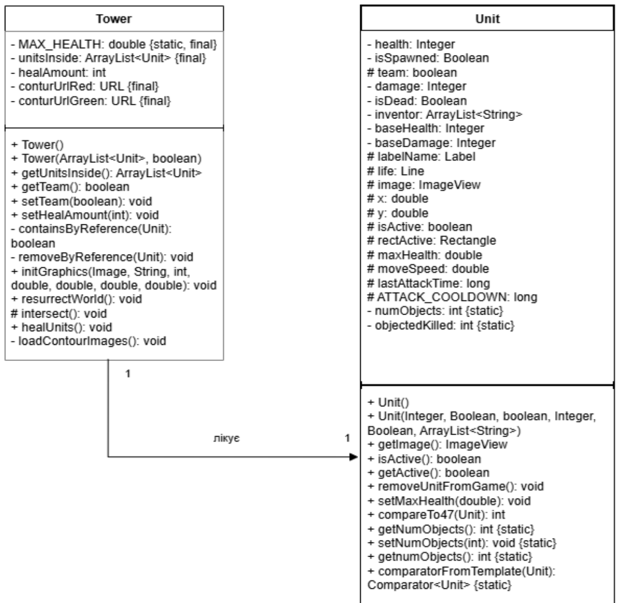
Рисунок 3.4 – Діаграма асоціації
