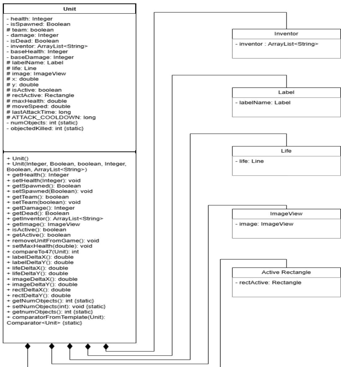
Рисунок 3.3 – Діаграма композиції
