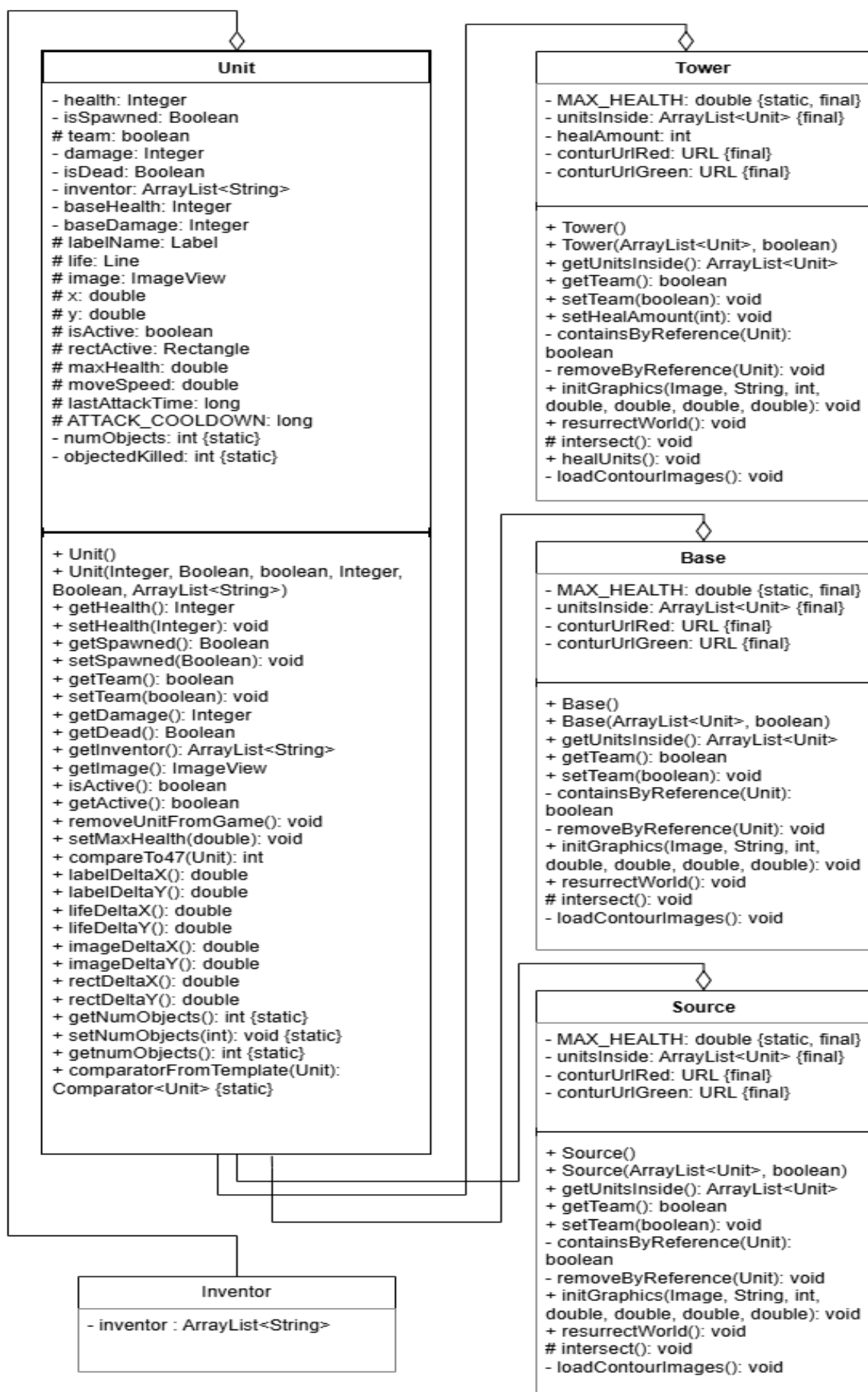
Рисунок 3.2 – Діаграма агрегації
