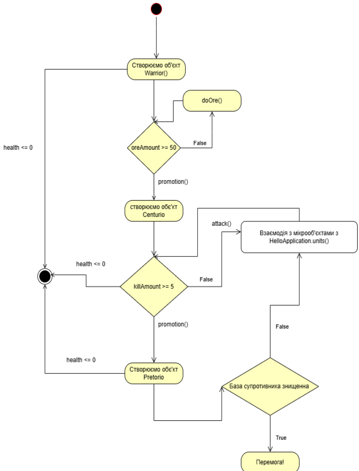
Рисунок 3.7 – Діаграма станів
