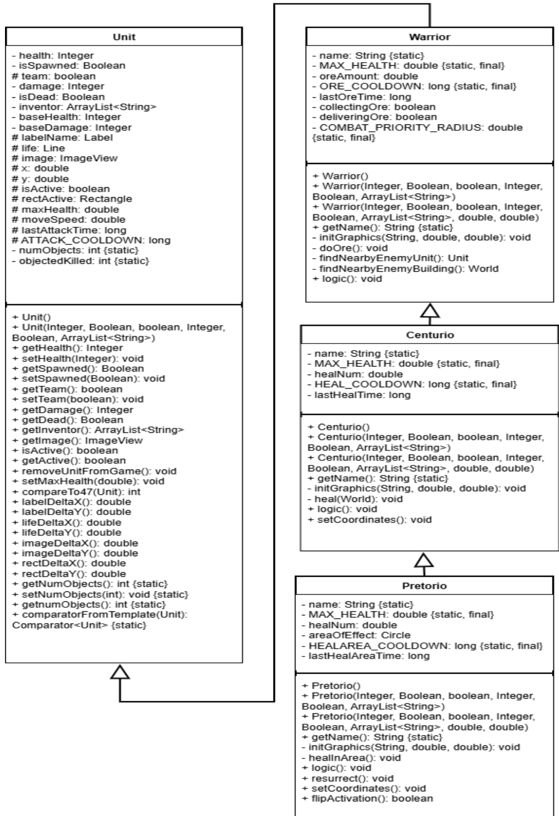
Рисунок 3.1 – Діаграма наслідування
